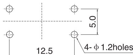
P.C.B.Land Pattern
