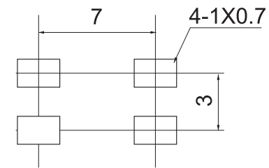
P.C.B.Land Pattern
