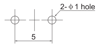
P.C.B. Land Pattern
