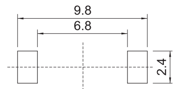
P.C.B.Land Pattern
